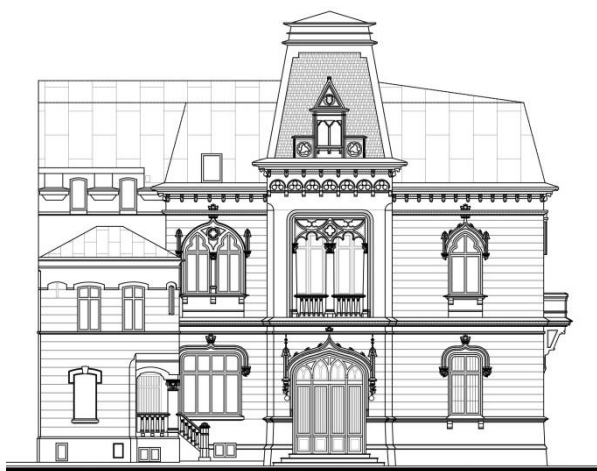
Casa Arhitecților (CCA al UAR) din Str. J. L. Calderon 48, relevu arh. Ioan și Adrian Crăciunescu
