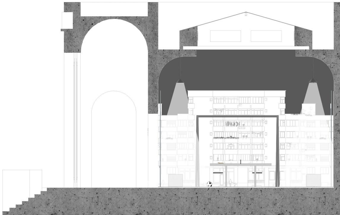
SECȚIUNE | SECTION 1:100
