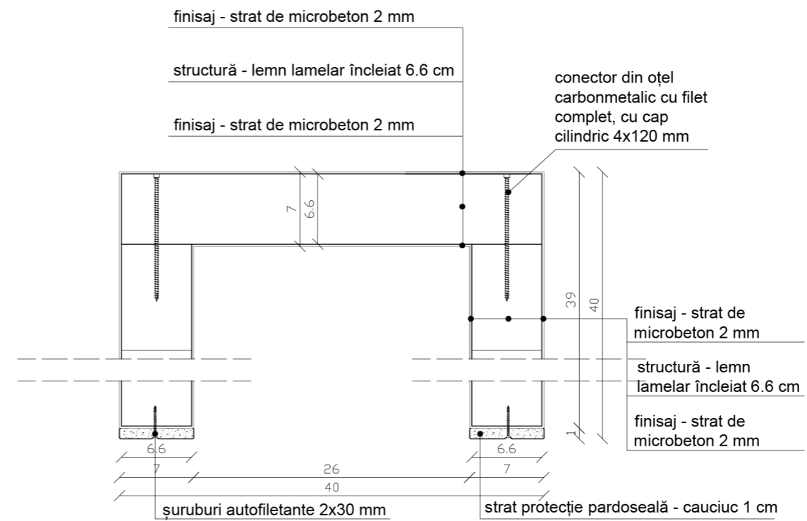
D2 - 1:5
