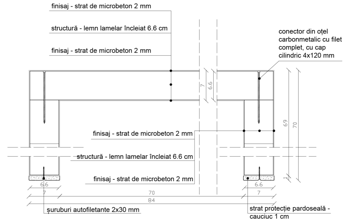
D1 - 1:5
