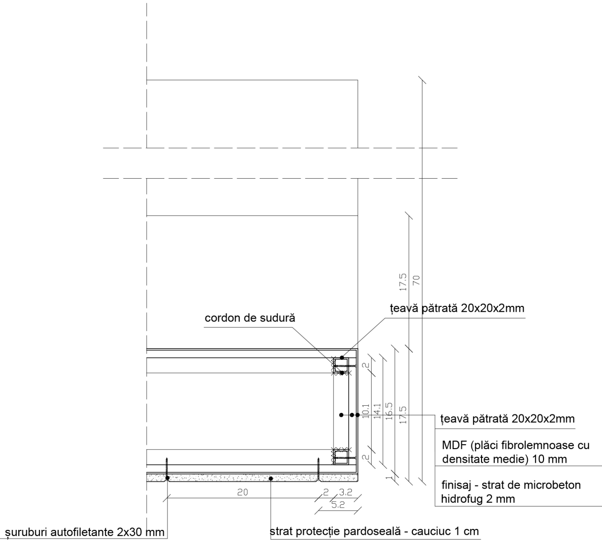
D1 - 1:5
