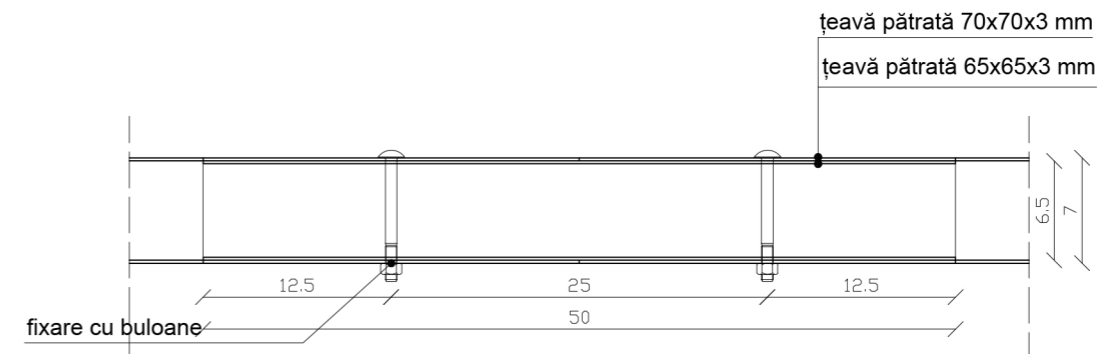
D2 - 1:5
