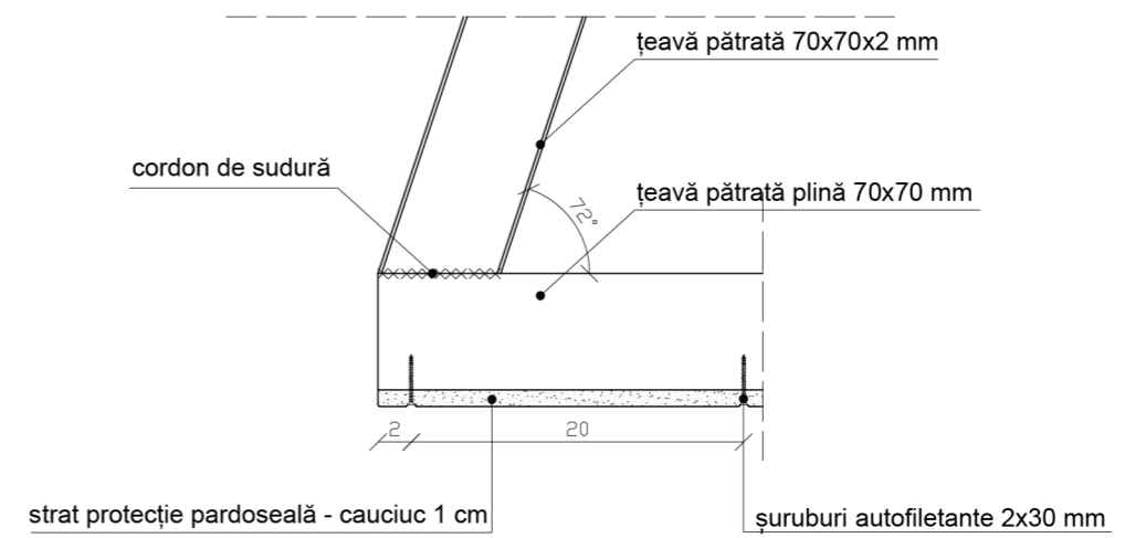
D3 - 1:5
