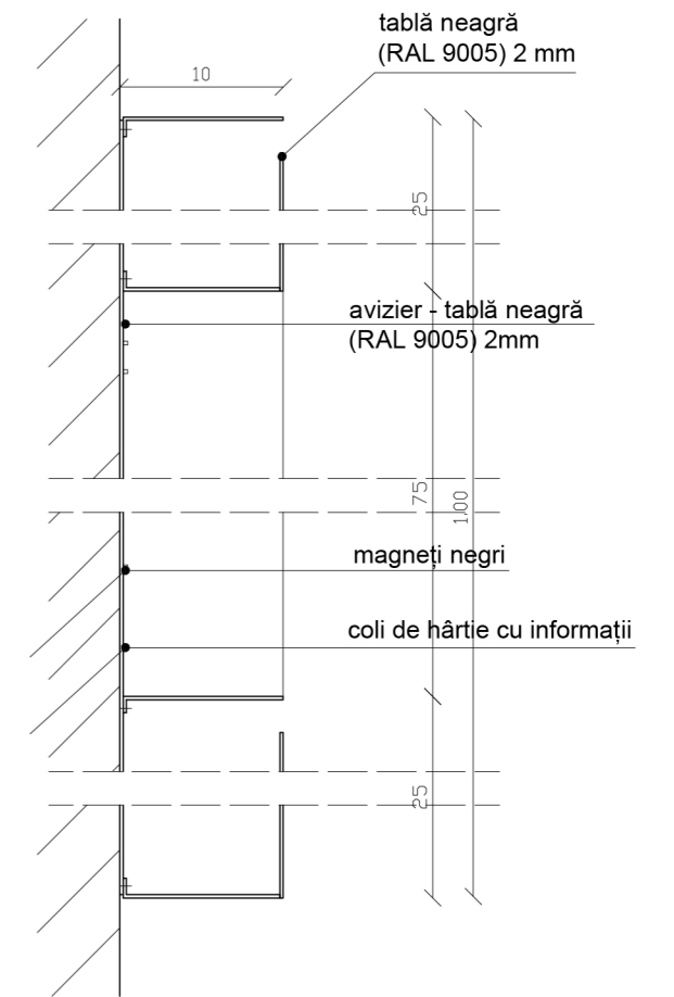
D3 - 1:5
