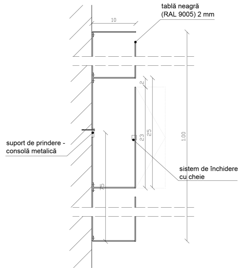
D2 - 1:5
